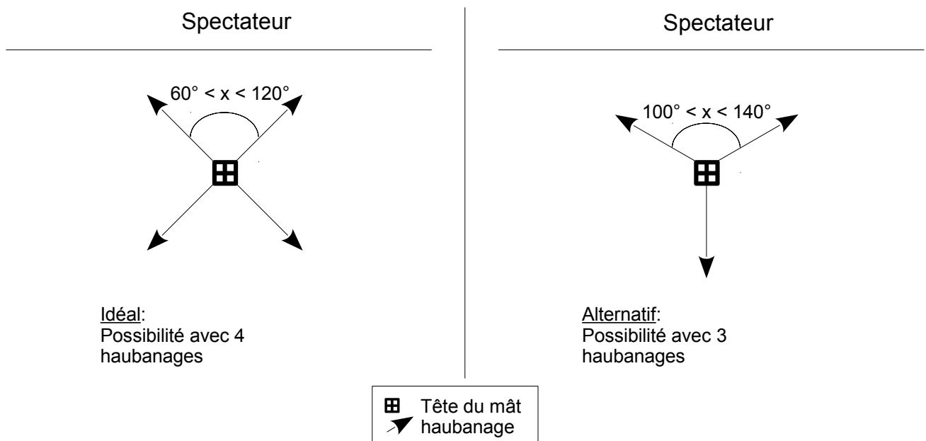
Vue d'en haut
